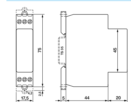
fig. 4. Dimensions (mm)
