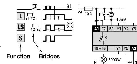
fig. 1. Wiring diagram
