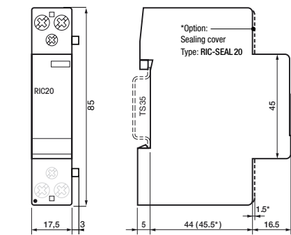
fig. 3. Dimensions (mm)
