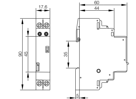
fig. 3. Dimensions (mm)
