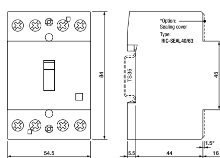
fig. 3. Dimensions (mm)
