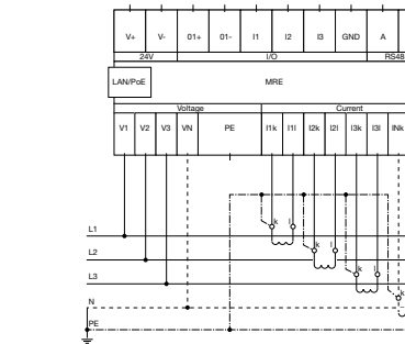
fig. 1. Wiring diagram
