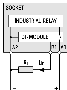
fig. 1. Wiring diagram
