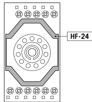
fig. 1. Dimensions (mm)
