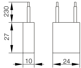
fig. 1. Dimensions (mm)
