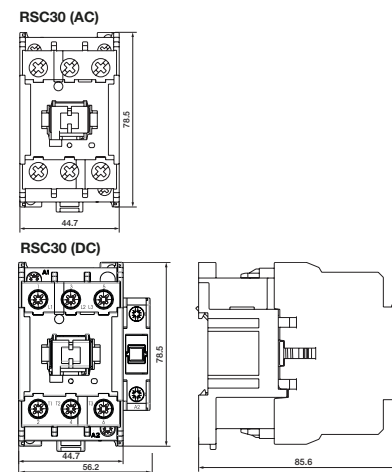
fig. 3. Dimensions (mm)
