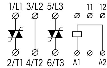
fig. 1. Wiring diagram
