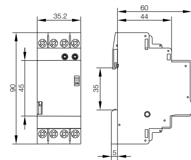
fig. 3. Dimensions (mm)
