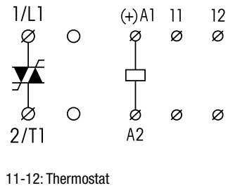
fig. 1. Wiring diagram
