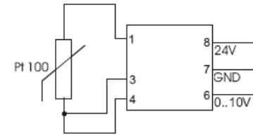
fig. 1. Wiring diagram
