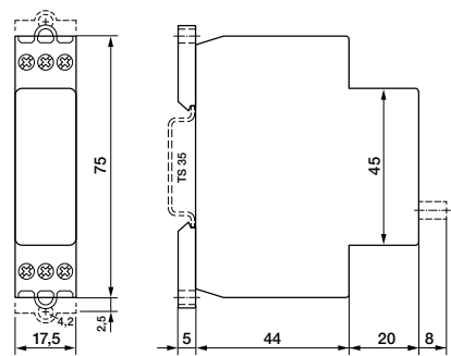
fig. 4. Dimensions (mm)
