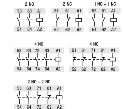
fig. 1. Wiring diagram
