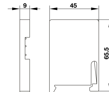
fig. 1. Dimensions (mm)
