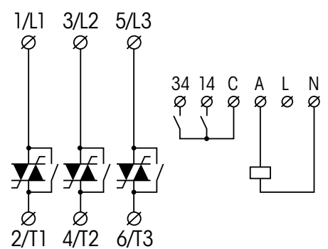
fig. 1. Wiring diagram
