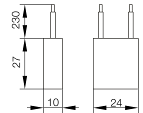
fig. 1. Dimensions (mm)
