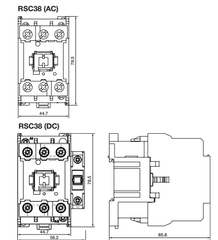
fig. 3. Dimensions (mm)
