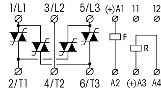
fig. 1. Wiring diagram
