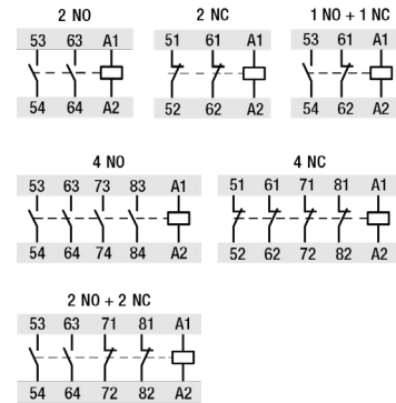
fig. 1. Wiring diagram
