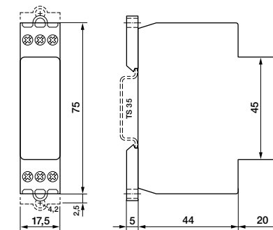
fig. 4. Dimensions (mm)
