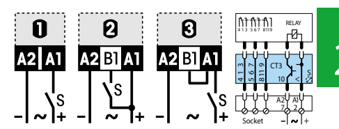
fig. 1. Wiring diagram
