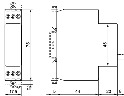
fig. 4. Dimensions (mm)
