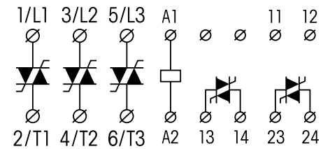
fig. 1. Wiring diagram
