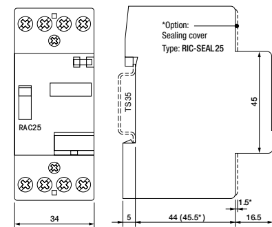
fig. 3. Dimensions (mm)
