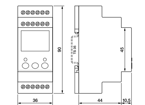
fig. 4. Dimensions (mm)
