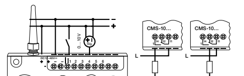
fig. 1. Wiring diagram
