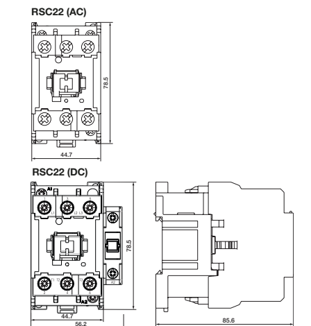
fig. 3. Dimensions (mm)
