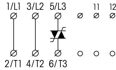
fig. 1. Wiring diagram
