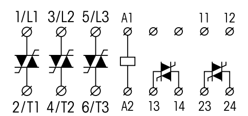
fig. 1. Wiring diagram
