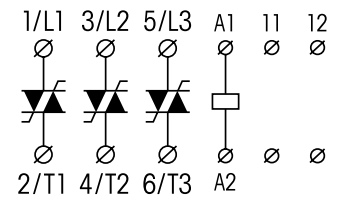
fig. 1. Wiring diagram
